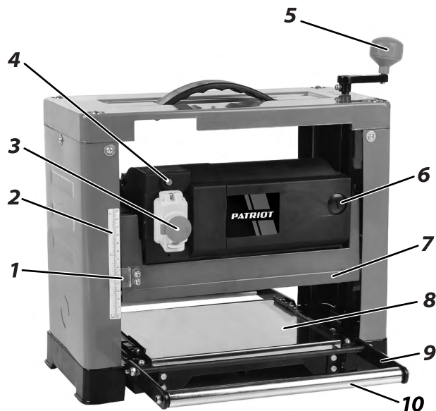
ВНЕШНИЙ ВИД ЭЛЕКТРОИНСТРУМЕНТА (Рис. 1)
